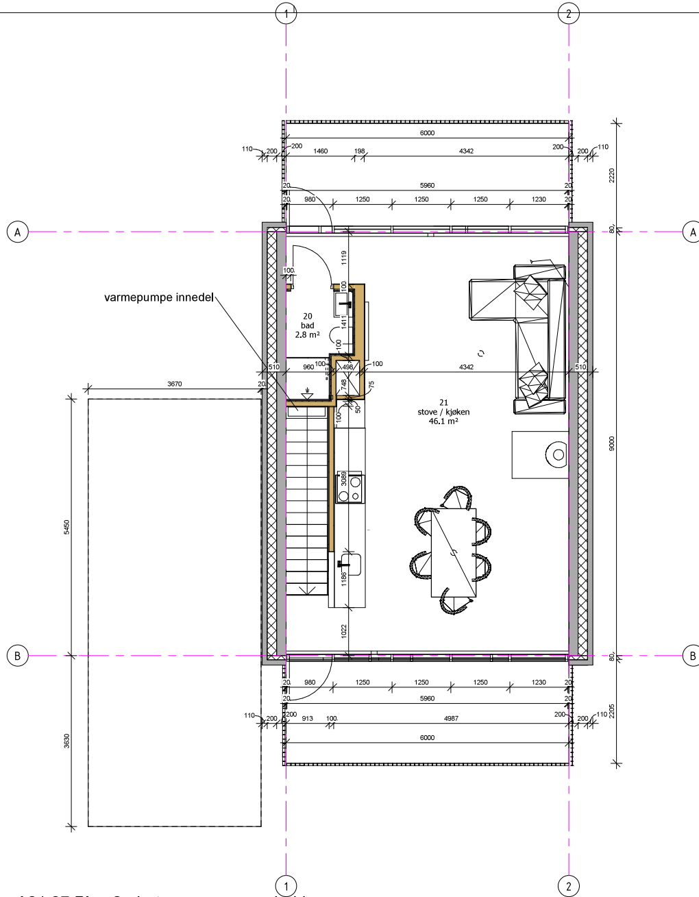
A21.27 Plan 2 - betong og grunnarbeid 1 : 50
